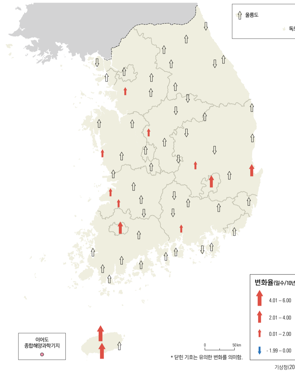
일 최저 기온 25°C 이상 연간일수 변화율(1973 - 2010년)
