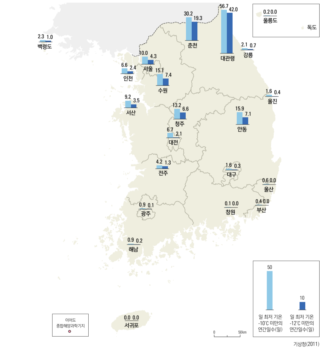
일 최저 기온 -10°C 미만의 연간일수와 일 최저 기온 -12°C 미만의 연간일수(1981 - 2010년)
