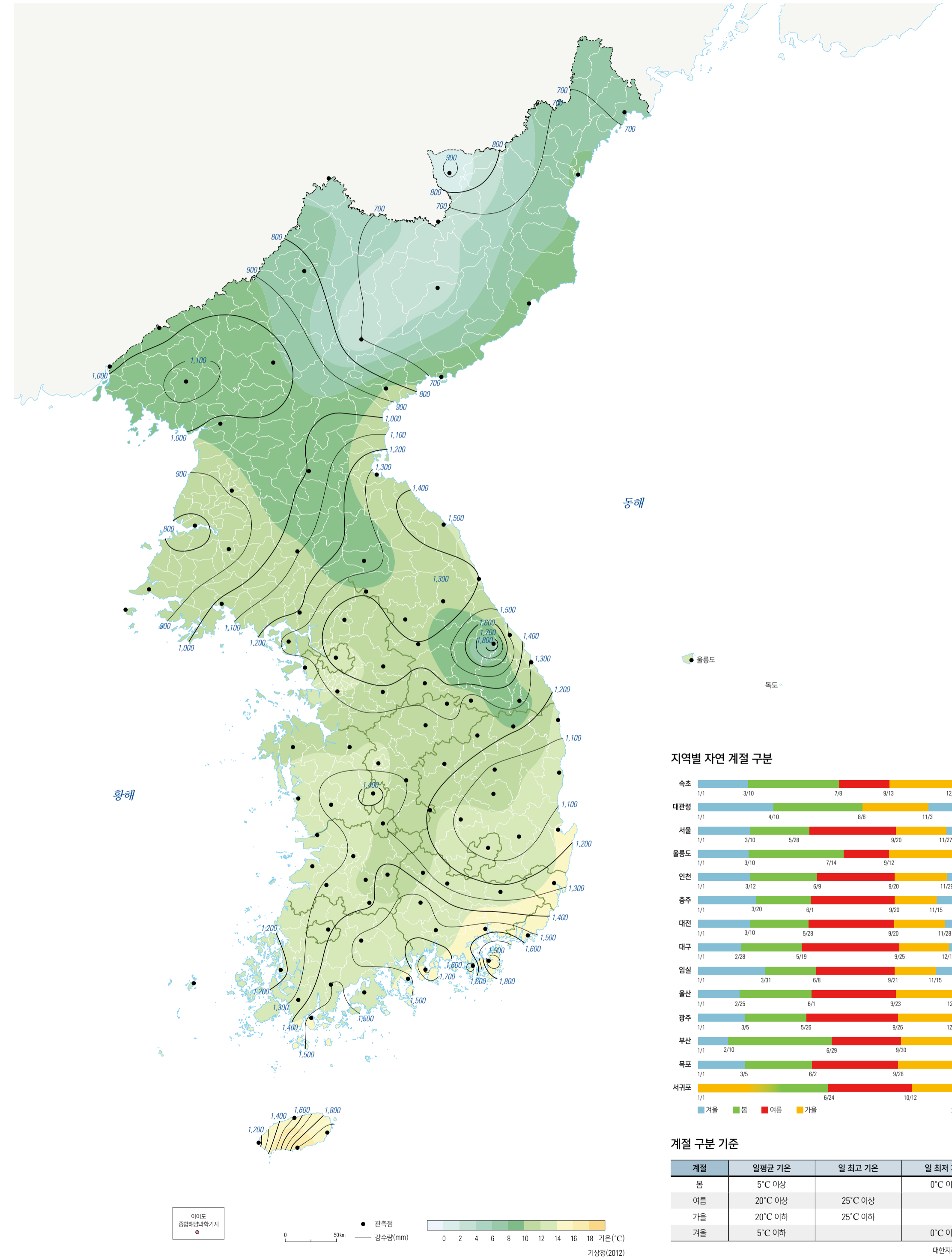
기후 개관 연평균 기온과 강수량
