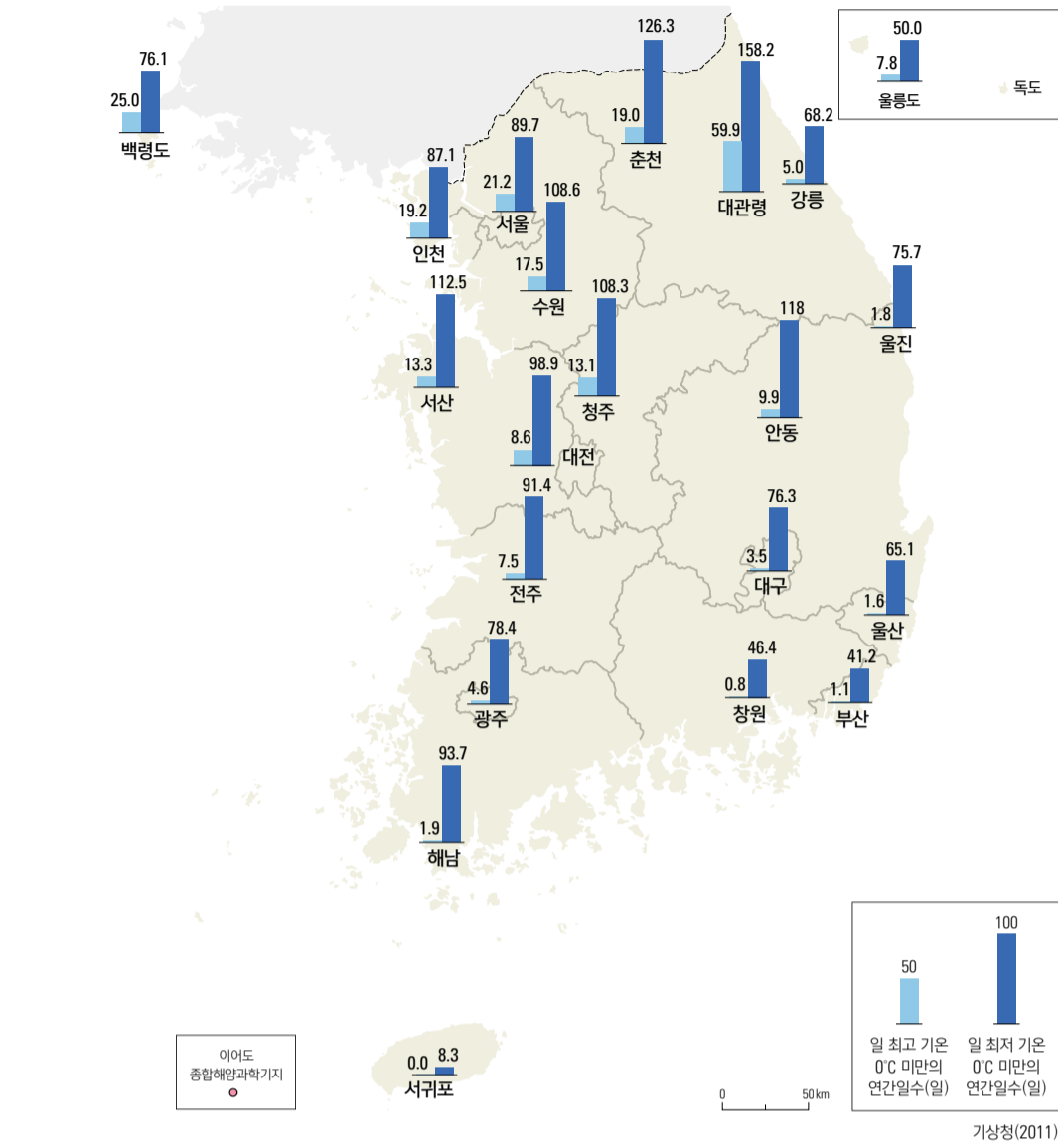
일 최고 기온 0°C 미만의 연간일수와 일 최저 기온 0°C 미만의 연간일수(1981 - 2010년)
