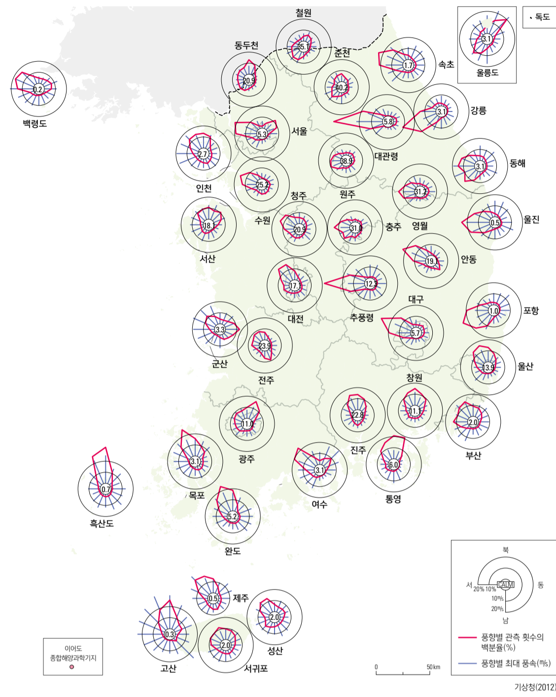
1월 바람장미(1981 - 2010년)
