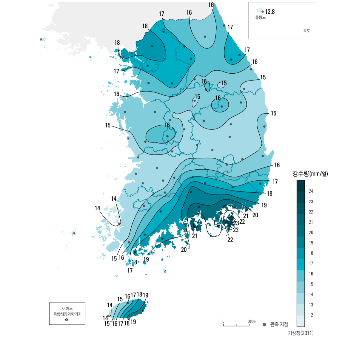
연 강수 강도(1981 - 2010년)
