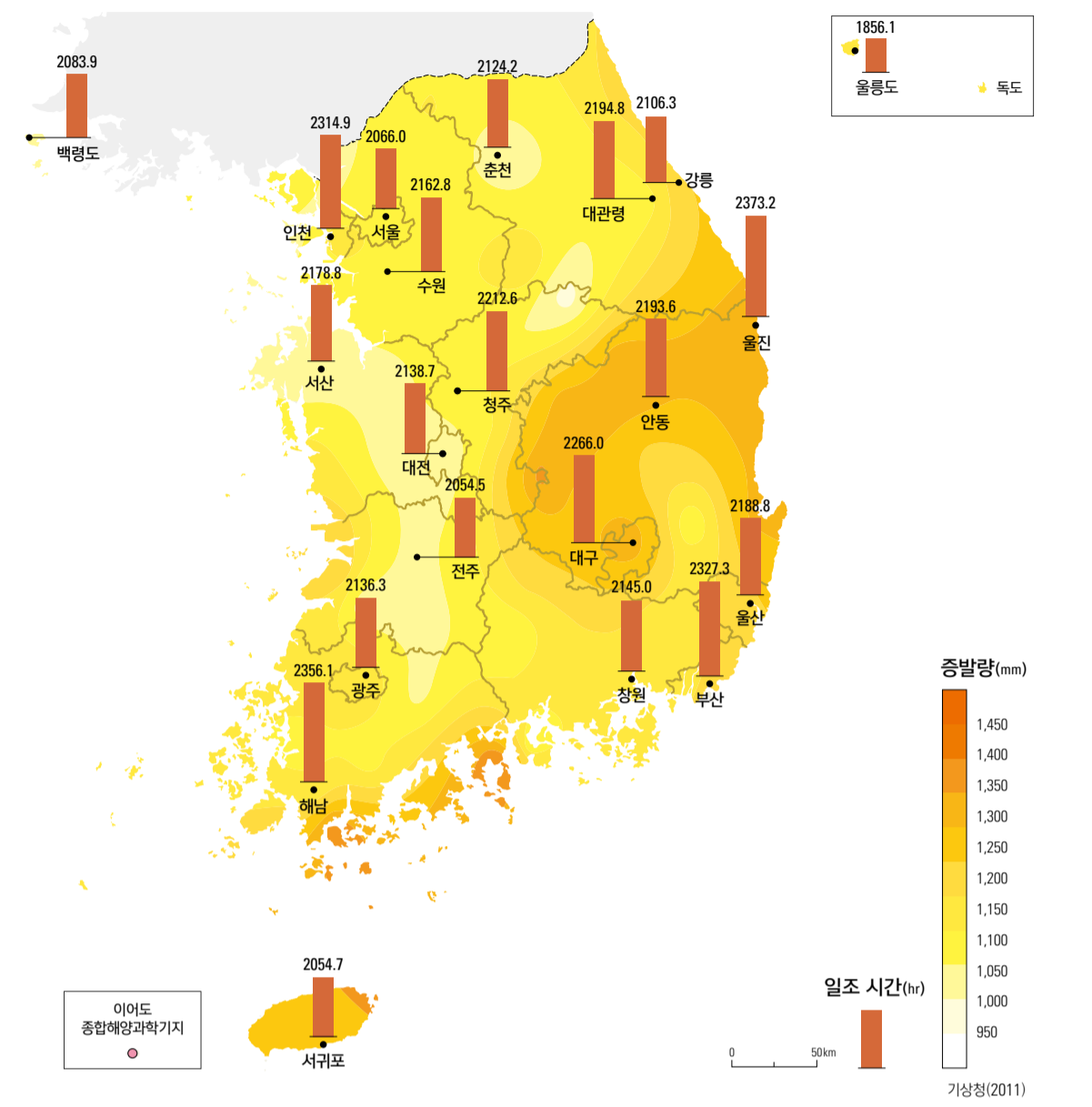
일조 시간과 연평균 증발량(1981 - 2010년)
