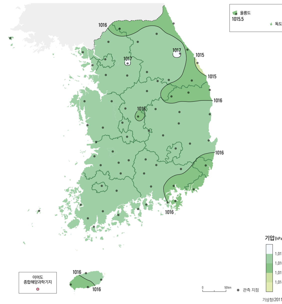
연평균 해면 기압(1981 - 2010년)
