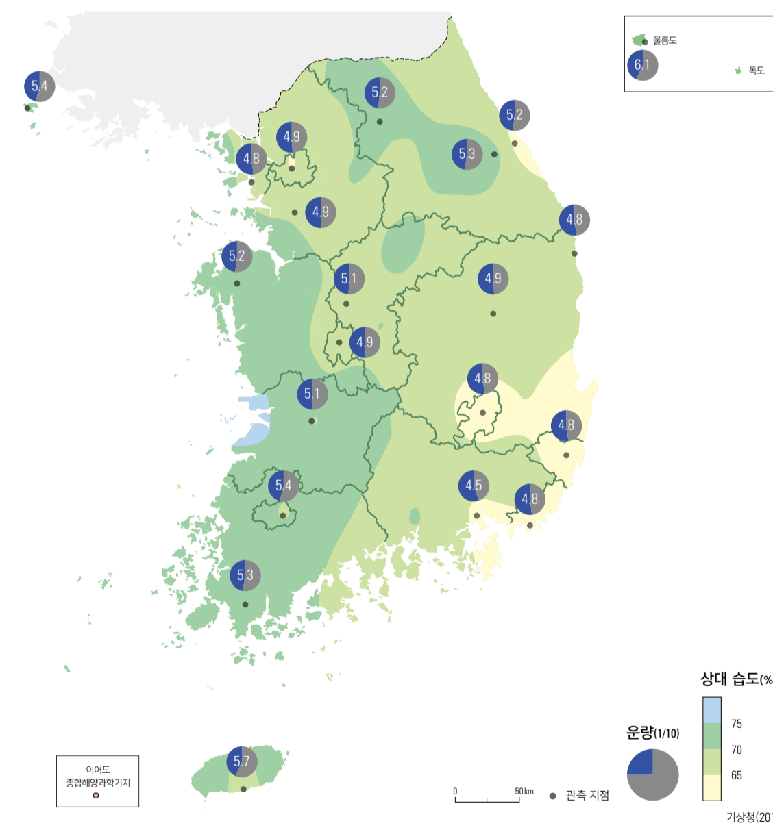
연평균 운량과 상대 습도(1981 - 2010년)
