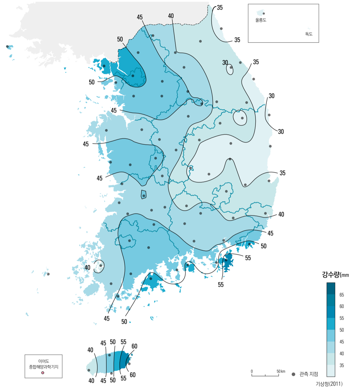
1시간 최대 강수량(1981 - 2010년)
