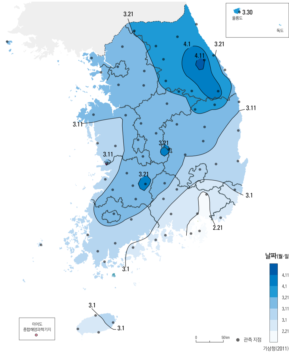
눈 마지막 날(1981 - 2010년)
