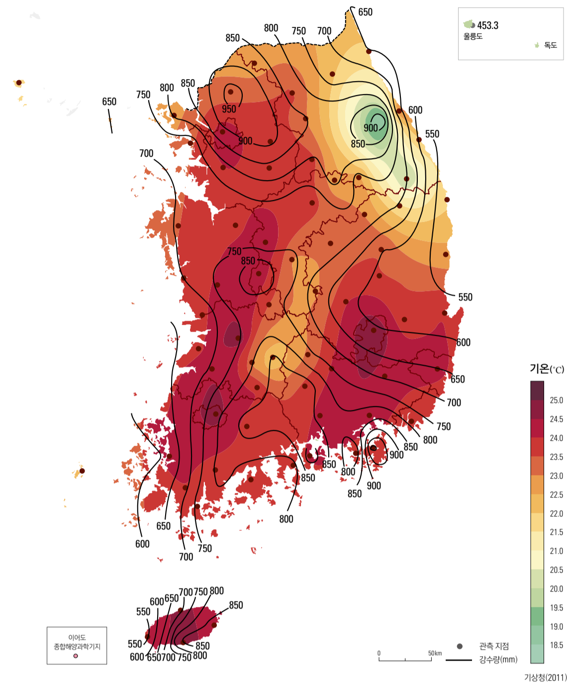
여름 평균 기온과 여름 강수량(1981 - 2010년)
