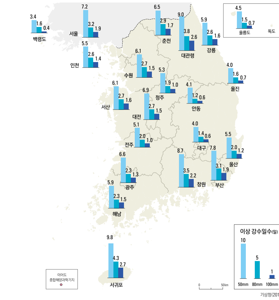
일 강수량 50mm, 80mm, 100mm 이상 일수(1981 - 2010년)
