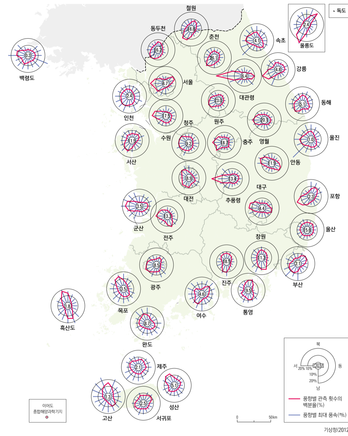
4월 바람장미(1981 - 2010년)
