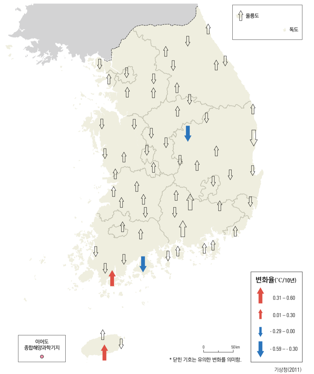
최고 기온 99퍼센타일 변화율(1973 - 2010년)
