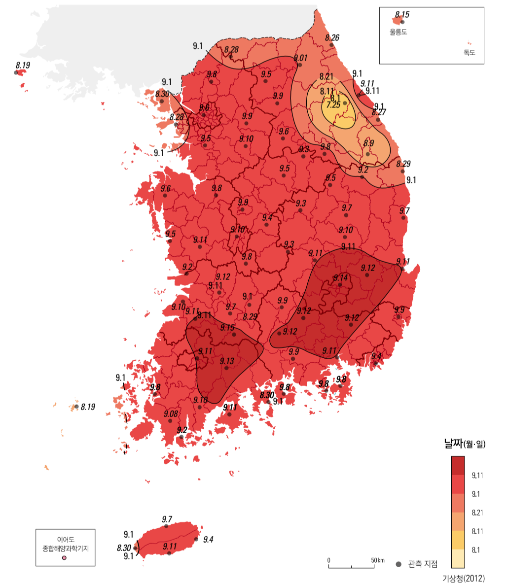
일 최고 기온 30°C 이상의 마지막 날(1981 - 2010년)
