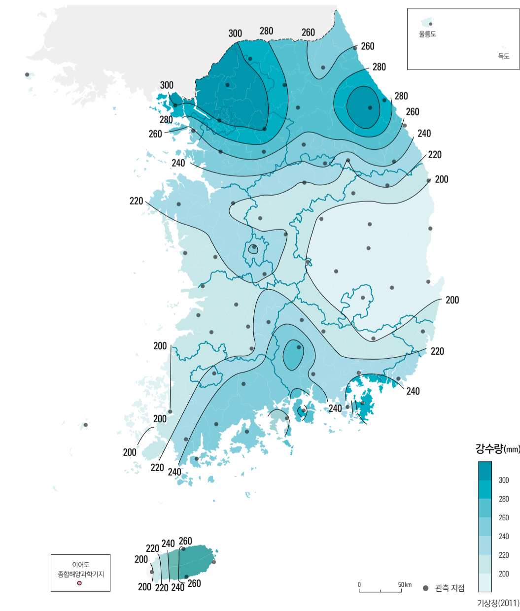
연 최대 5일 연속 강수량(1981 - 2010년)
