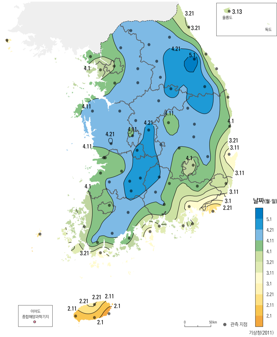
서리 마지막 날(1981 - 2010년)
