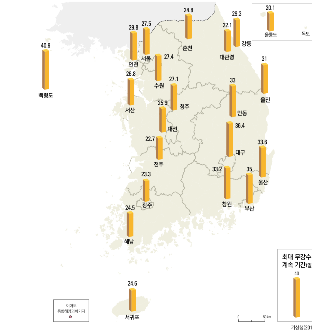
최대 무강수 계속 기간(1981 - 2010년)
