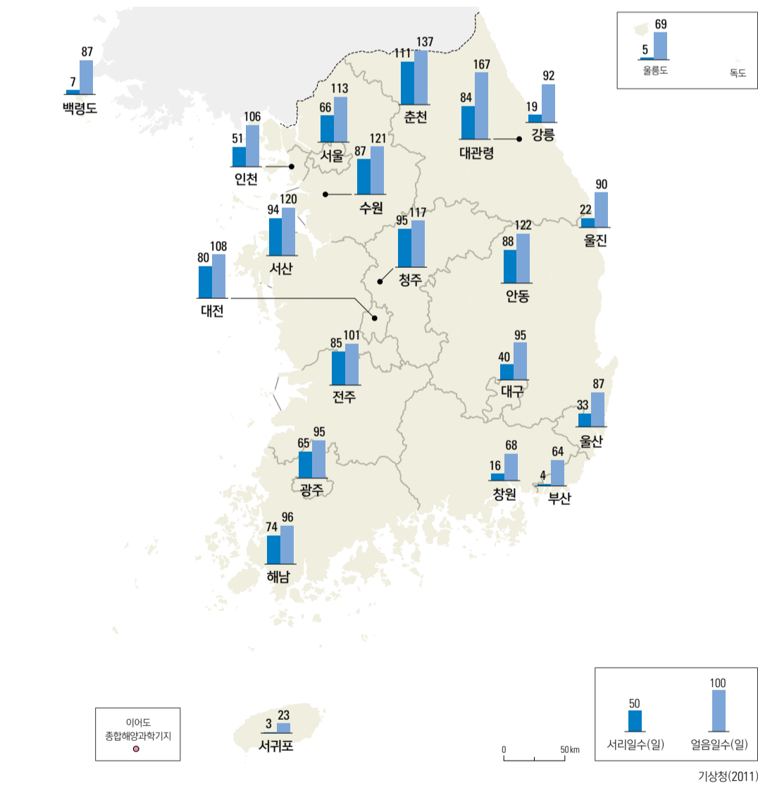
연 서리일수와 연 얼음일수(1981 - 2010년)
