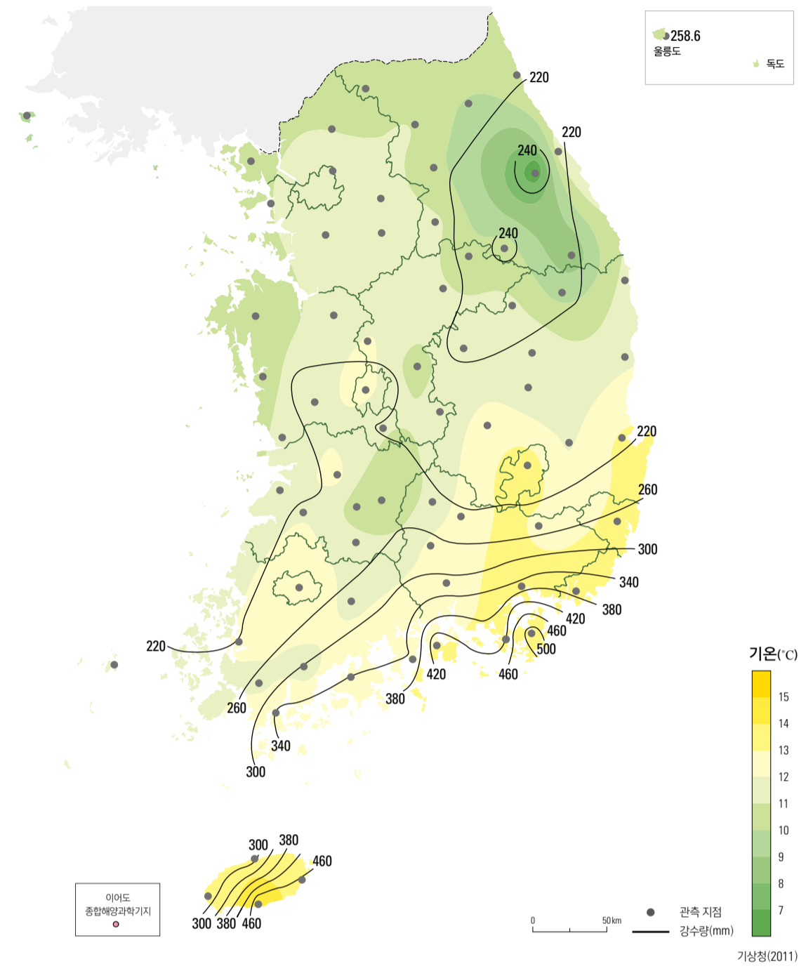
봄 평균 기온과 봄 강수량(1981 - 2010년)
