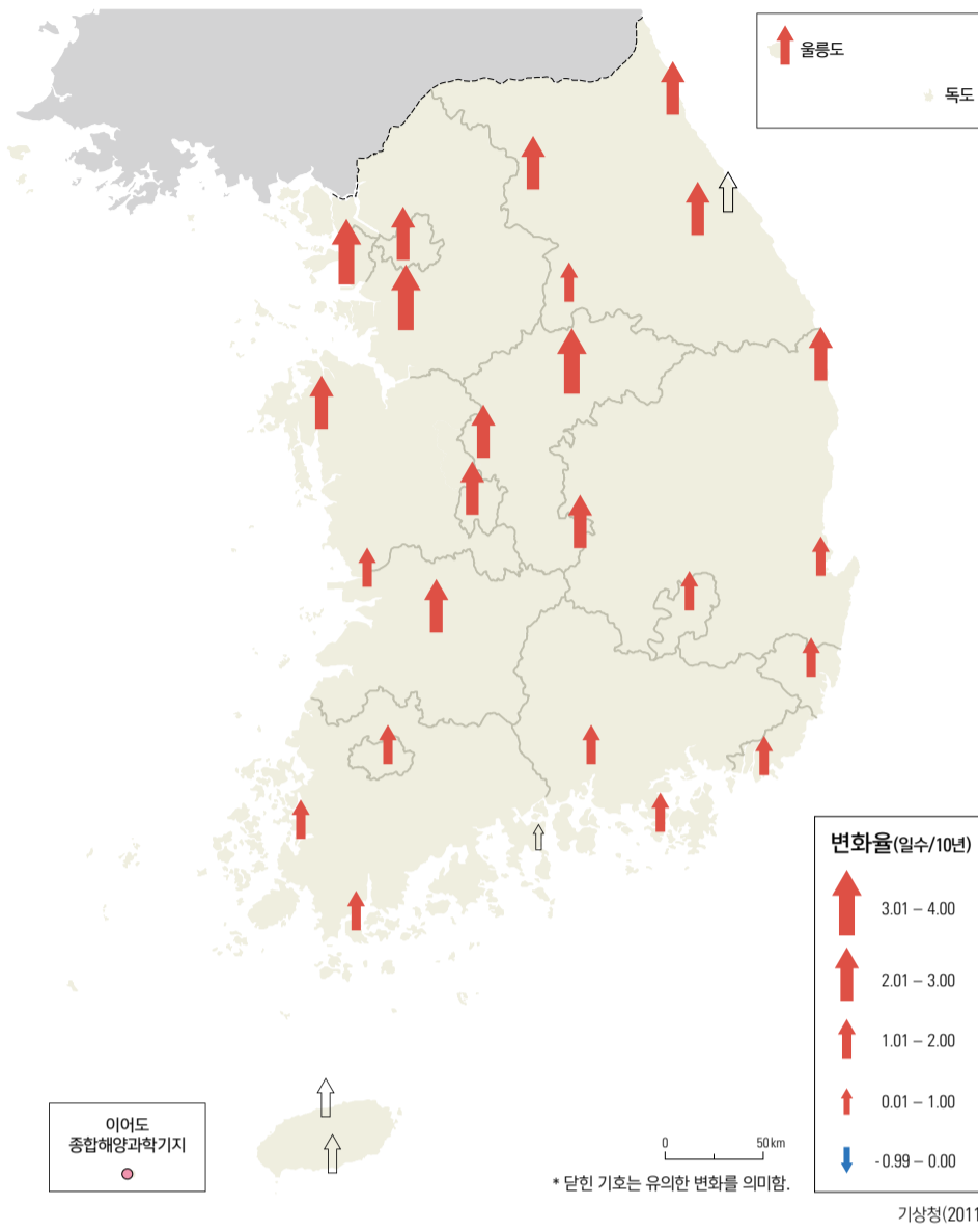
연 황사일수 변화율(1973 - 2010년)
