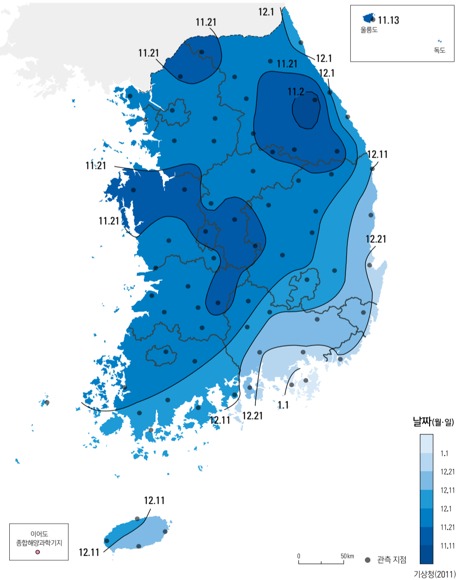
눈 첫날(1981 - 2010년)
