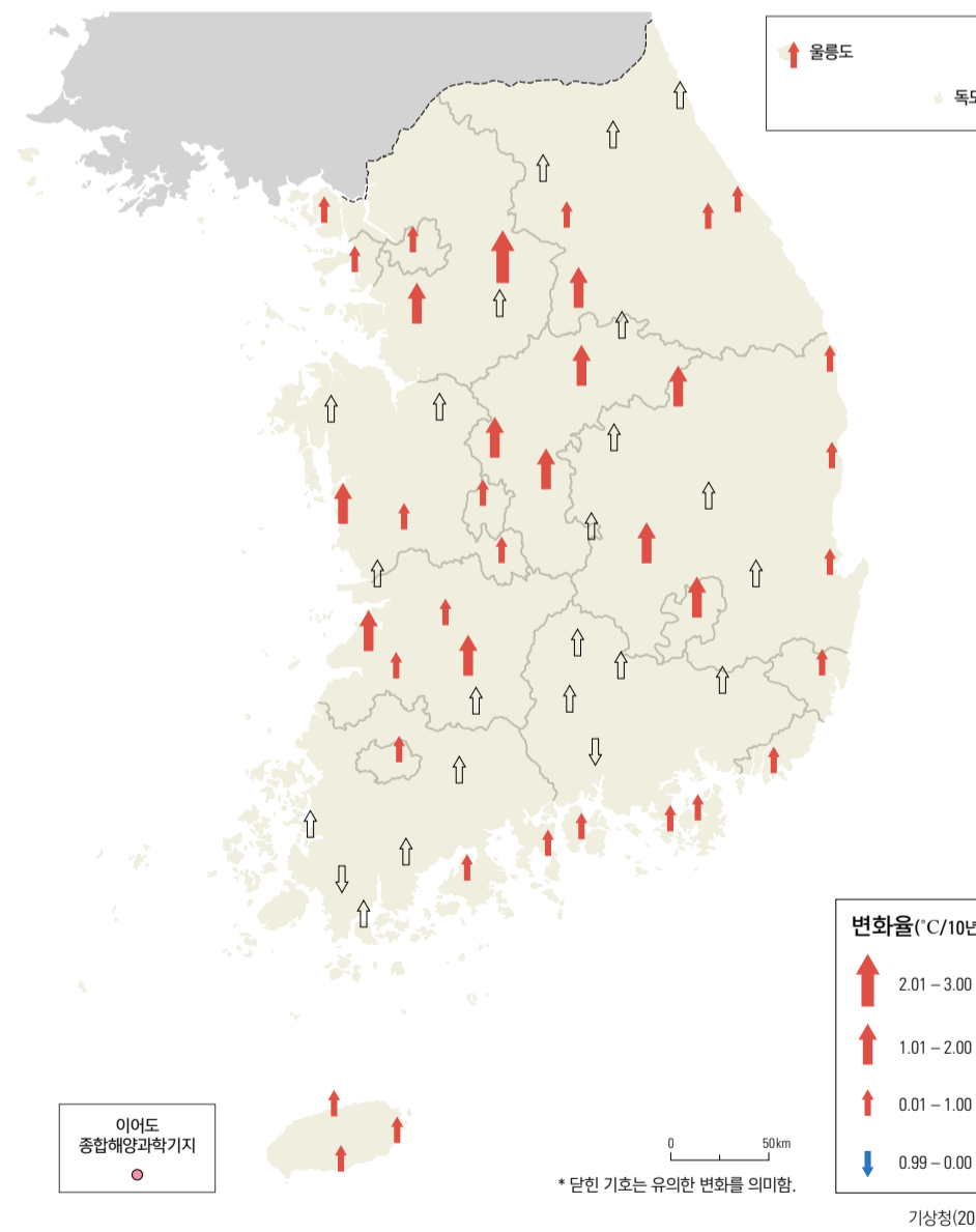
최저 기온 1퍼센타일 변화율(1973 - 2010년)
