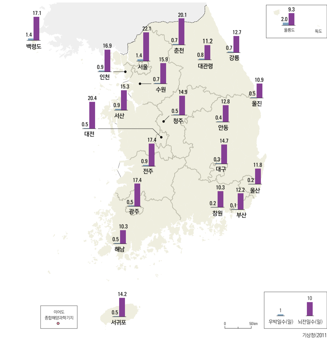
연 우박일수와 연 뇌전일수(1981 - 2010년)
