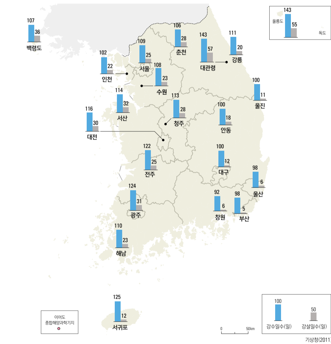
연 강수일수와 연 강설일수(1981 - 2010년)
