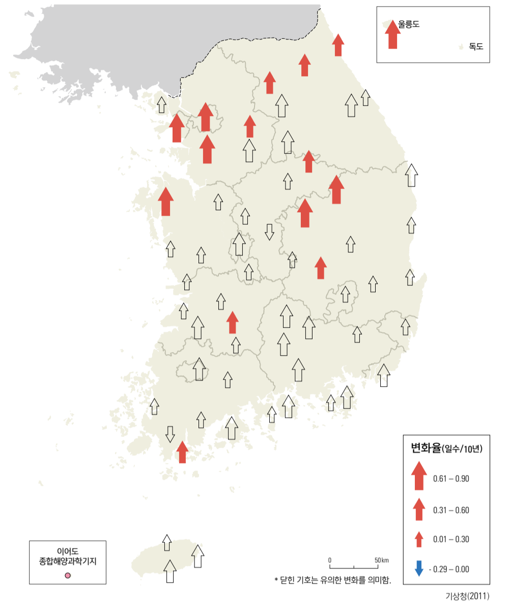
일 강수량 80mm 이상 연간일수 변화율(1973 - 2010년)
