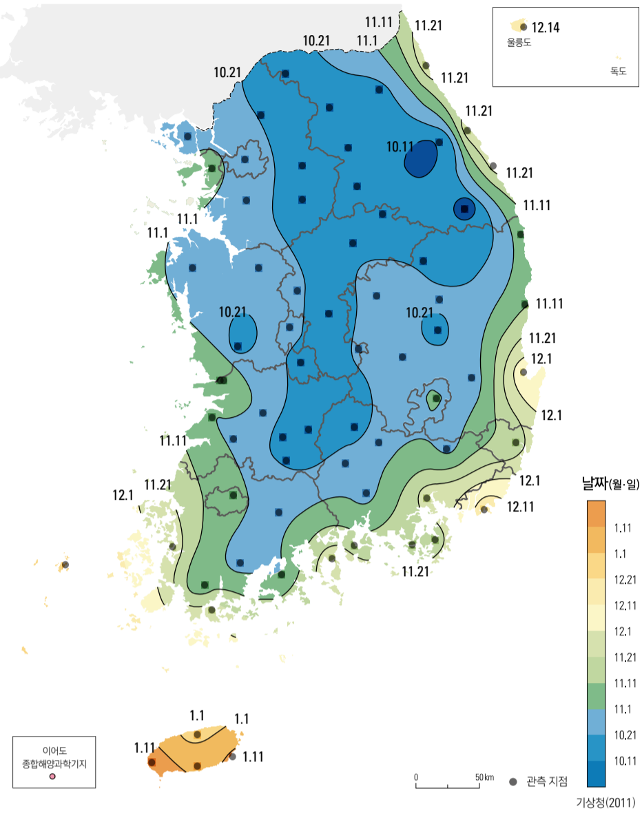
서리 첫날(1981 - 2010년)
