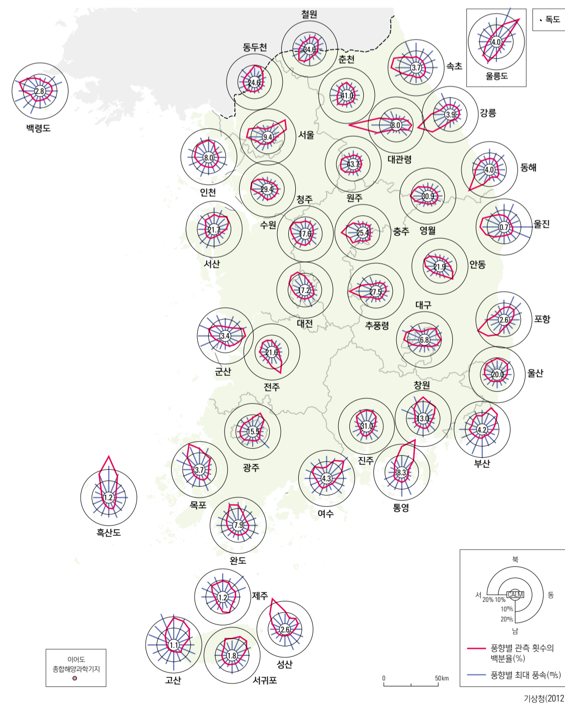
10월 바람장미(1981 - 2010년)
