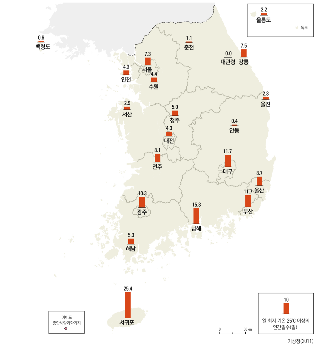
일 최저 기온 25°C 이상의 연간일수(1981 - 2010년)
