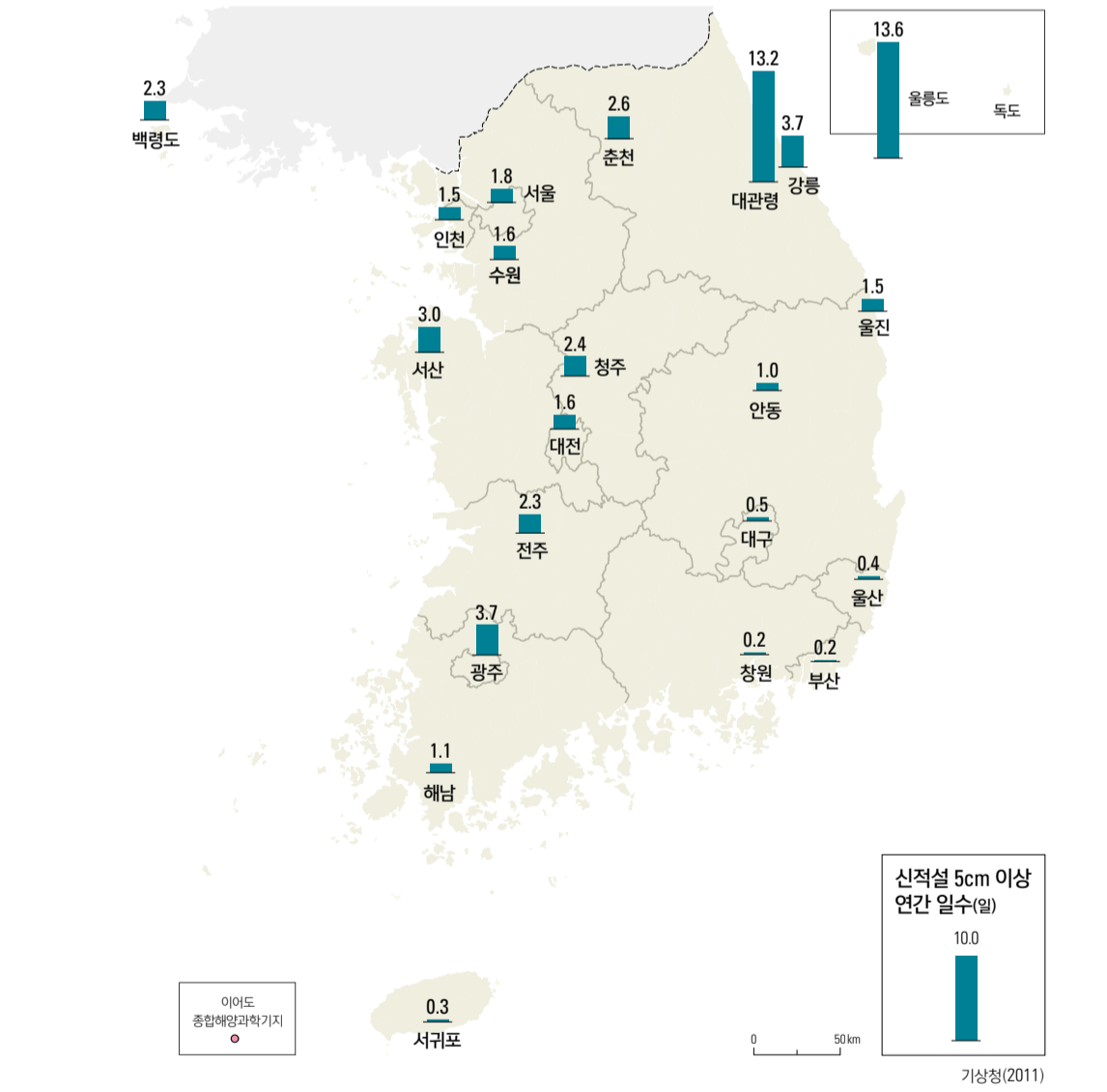
신적설 5cm 이상 연간일수(1981 - 2010년)
