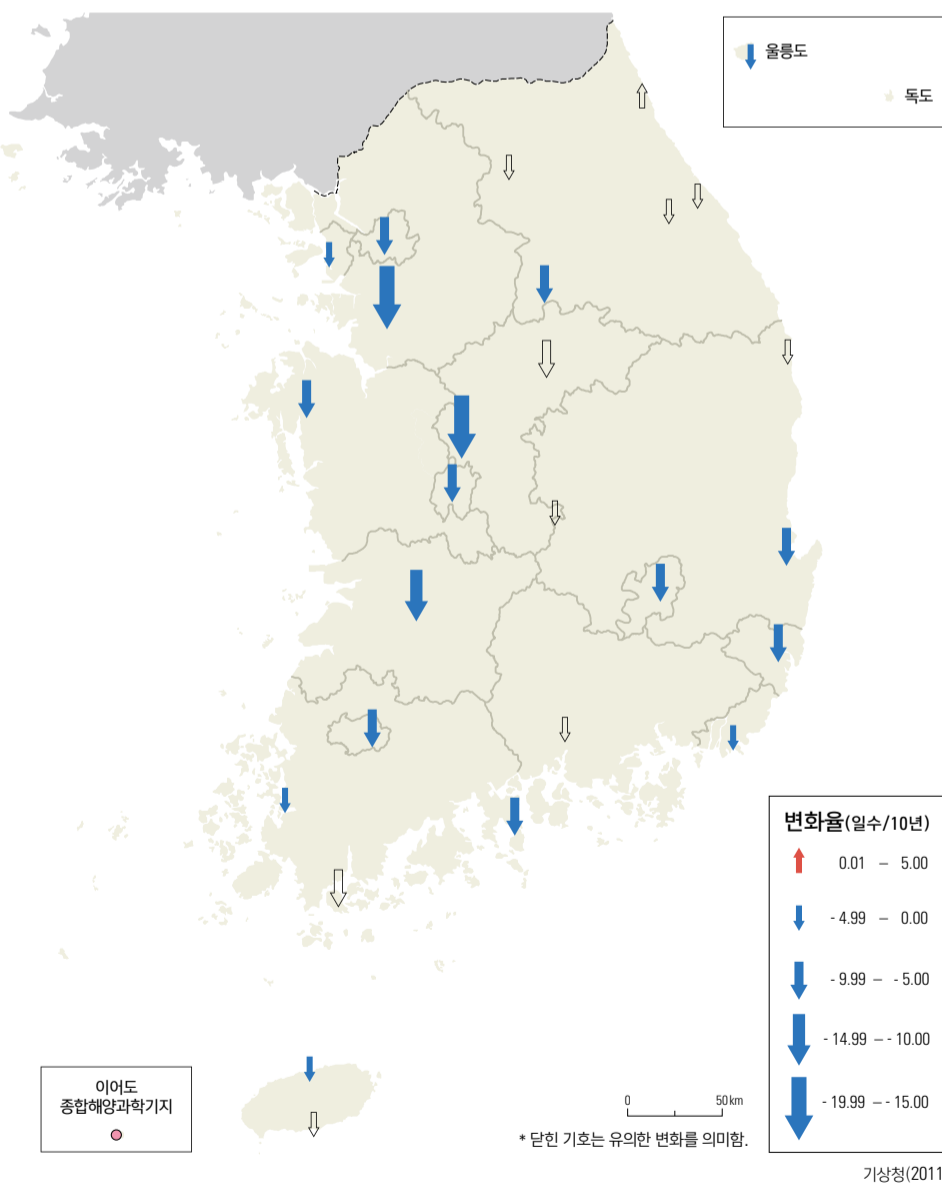
연 서리일수 변화율(1973 - 2010년)
