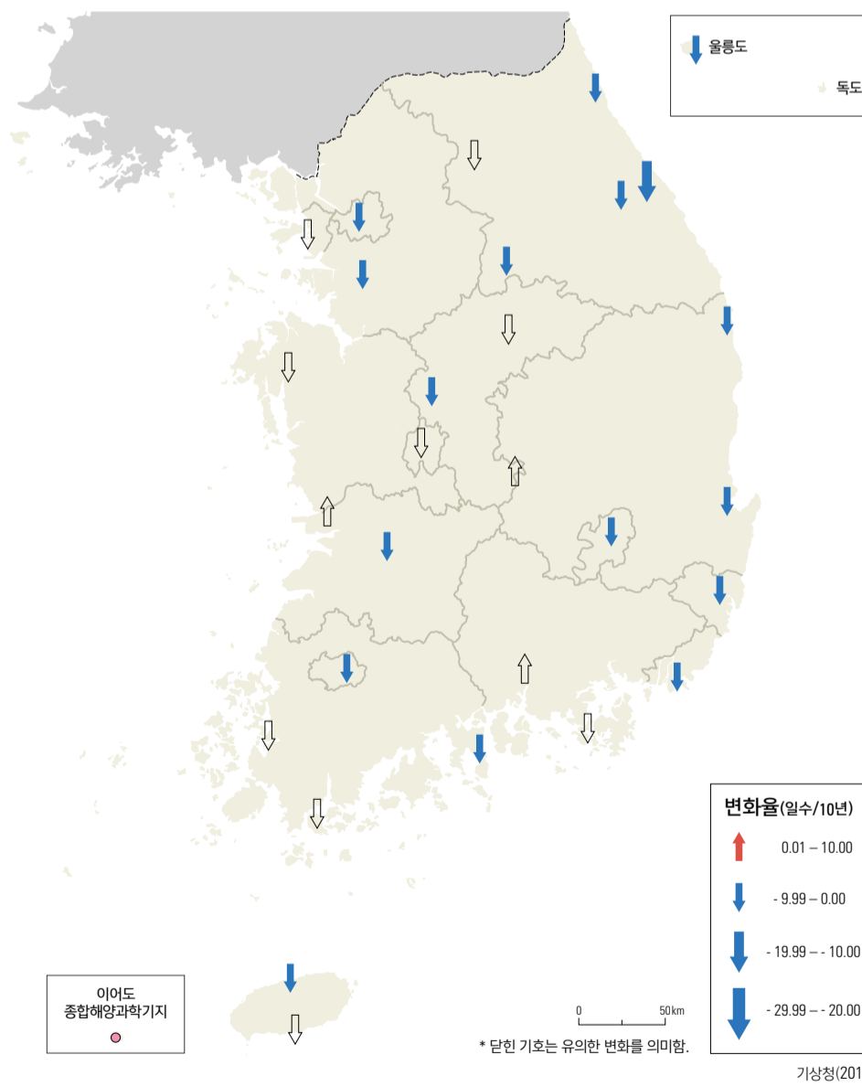
연 얼음일수 변화율(1973 - 2010년)
