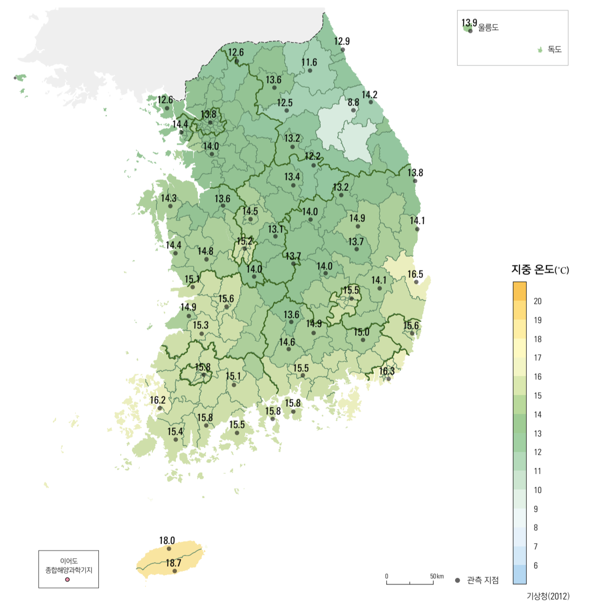
시·군별 연평균 지중 온도(1981 - 2010년)
