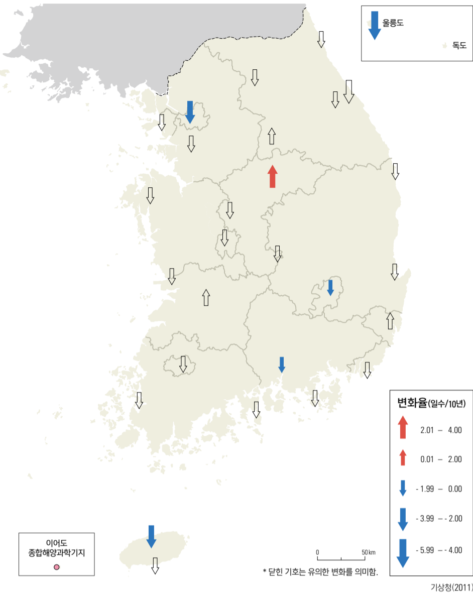
연 눈일수 변화율(1973 - 2010년)
