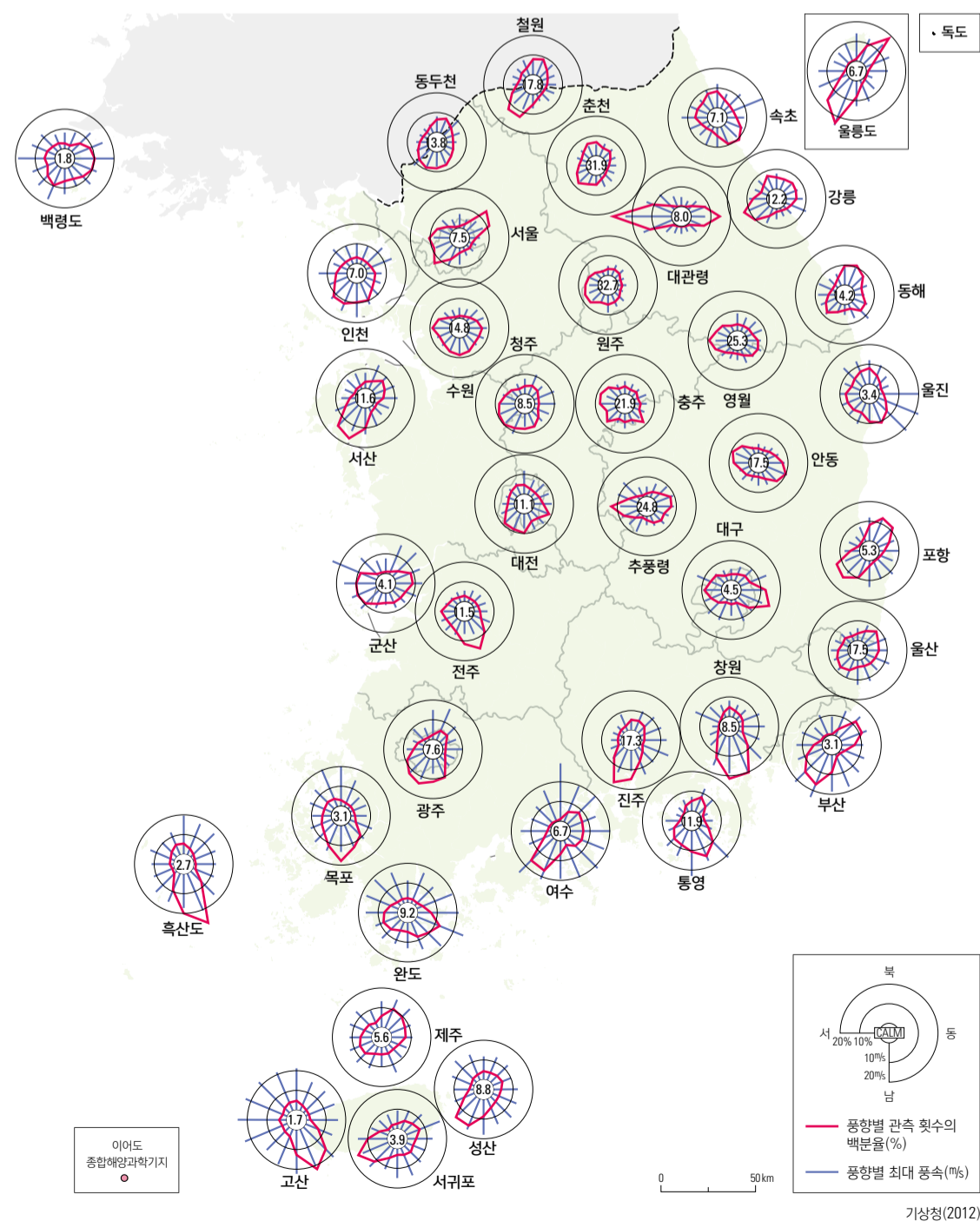
7월 바람장미(1981 - 2010년)
