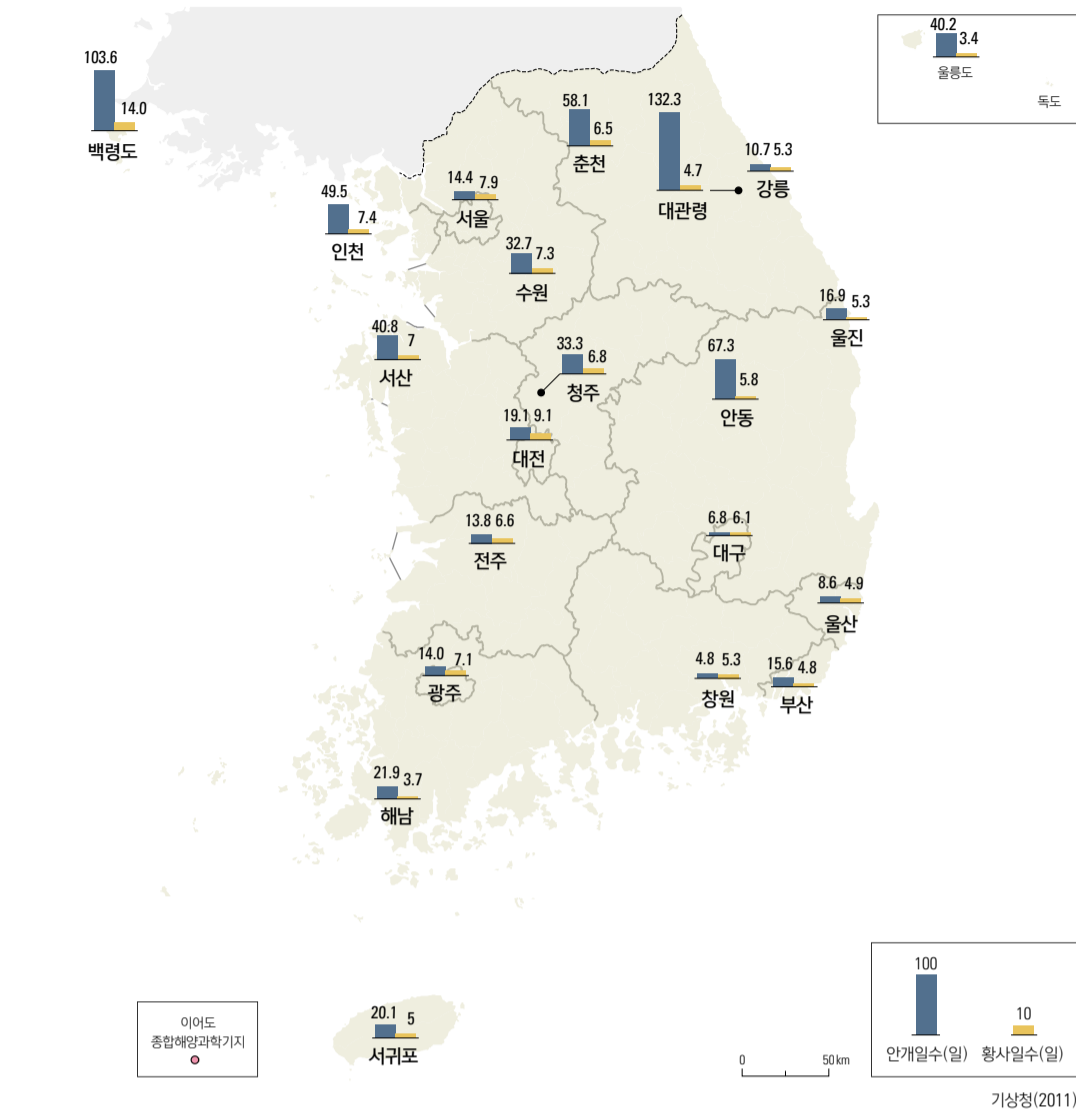
연 안개일수와 연 황사일수(1981 - 2010년)
