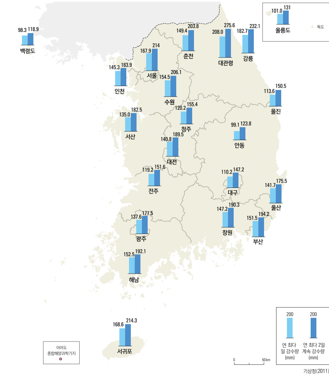
연 최대 일 강수량과 연 최대 2일 연속 강수량(1981 - 2010년)
