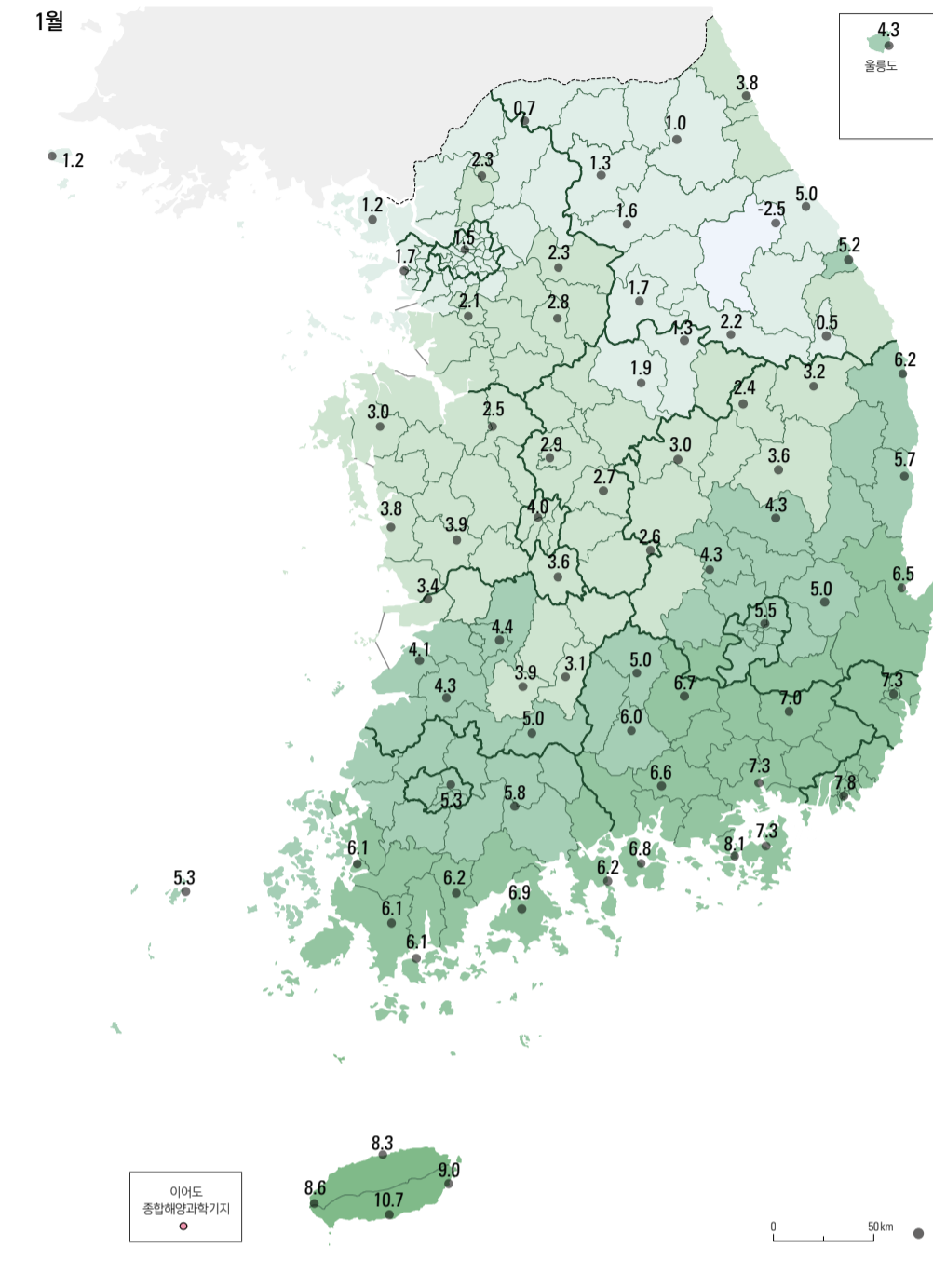
시·군별 월 평균 최고 기온(1981 - 2010년)
