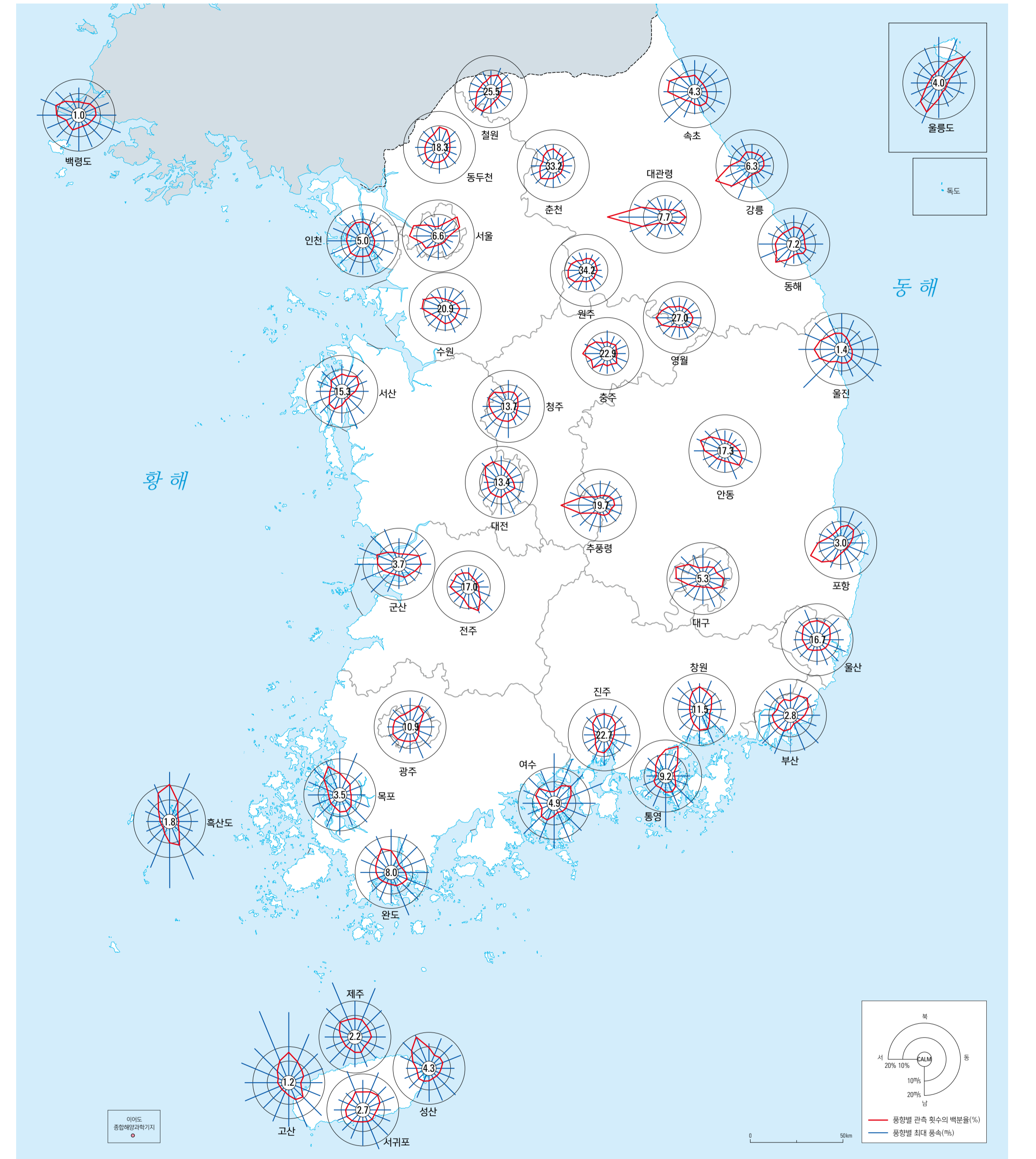
관측 지점별 연평균 바람장미(1981 - 2010년)
