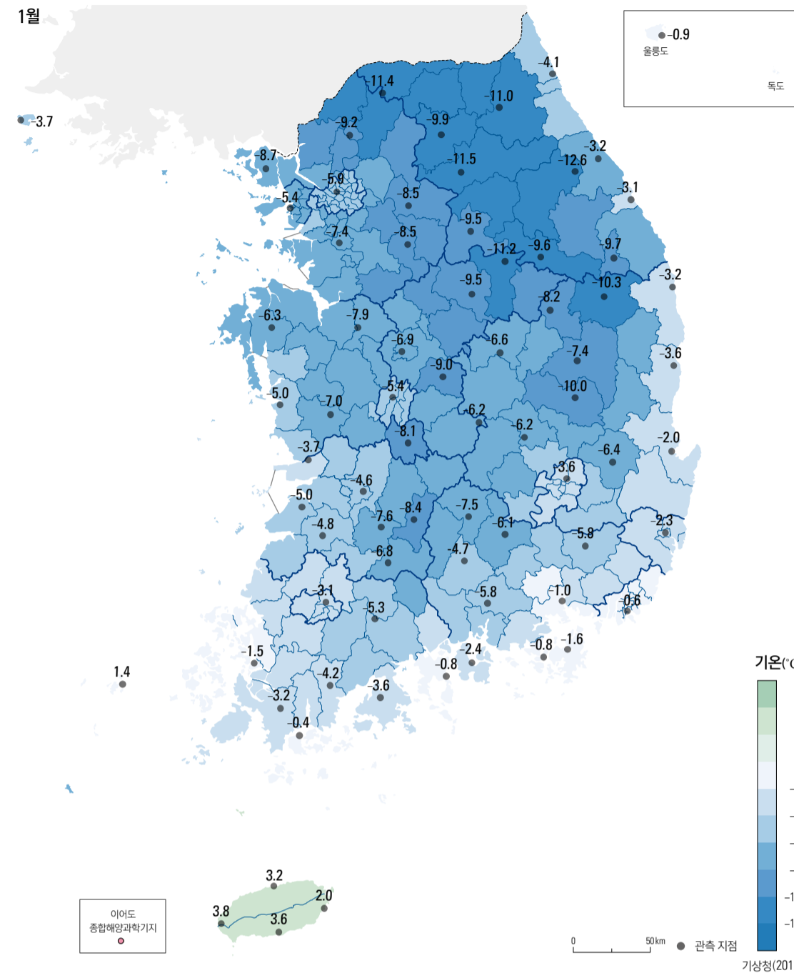
시·군별 월평균 최저 기온(1981 - 2010년)
